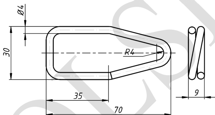
Рисунок 1. Карабин для зажима ODWAC
