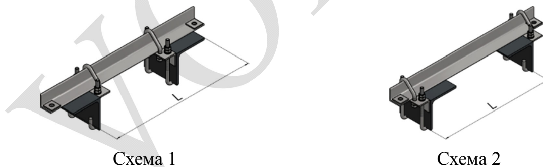
Рисунок 2. Способ крепления
