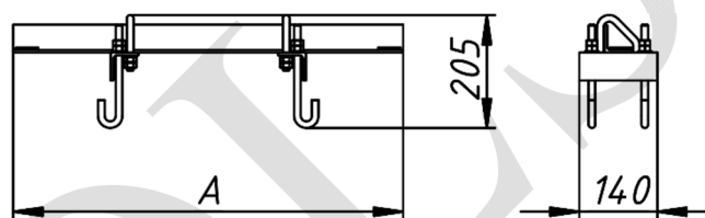
Рисунок 1. Узел натяжной УН(3)
