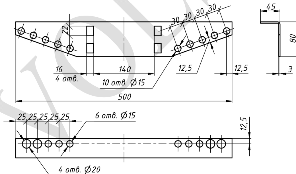
Рисунок 1. Траверса СТ8У
