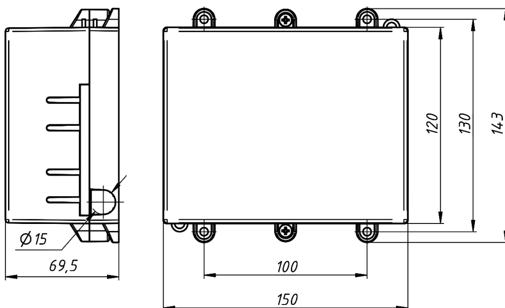
Рисунок 1. Габаритные размеры. Оптическая кросс-муфта ОКМ-П-16С/8С
