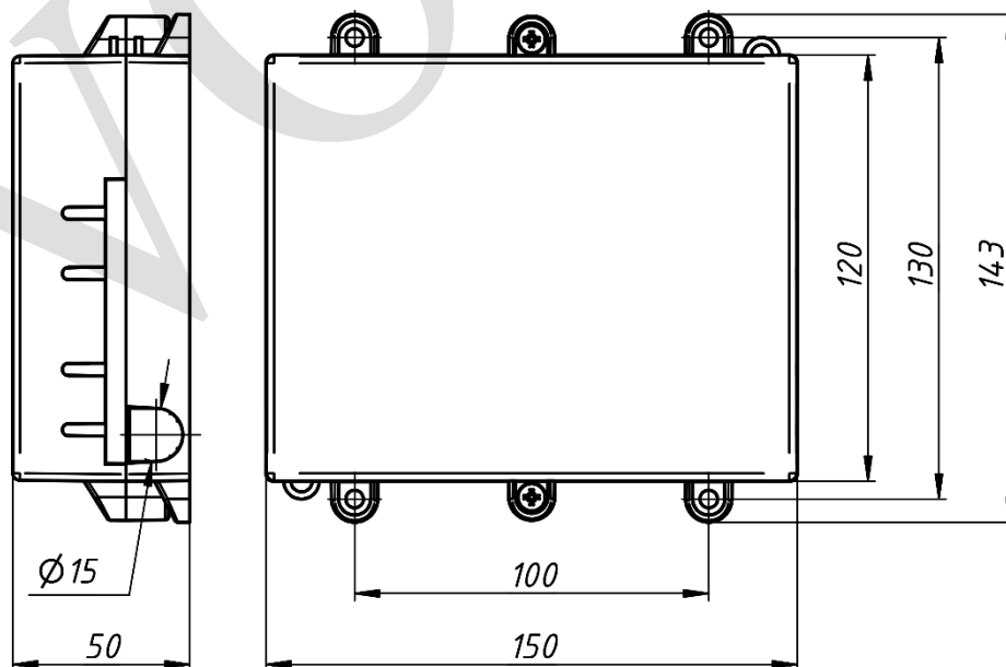
Рисунок 1. Оптическая кросс-муфта ОКМ-1513-4-SC/APC
