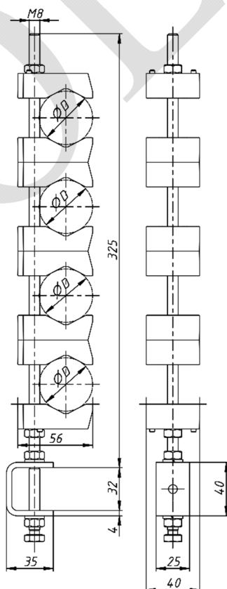
Рисунок 1. Зажим на четыре кабеля диаметр 24-29 мм
