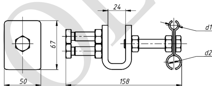
Рисунок 1. Зажим шлейфовый ЗКШ2-М 18/20-4
