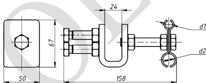
Рисунок 1. Зажим шлейфовый ЗКШ2-М 11/14-2
