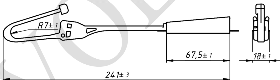
Рисунок 1. Зажим анкерный VS-O-НУ
