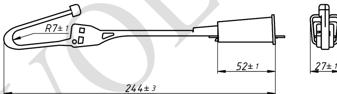
Рисунок 1. Зажим анкерный Р-25
