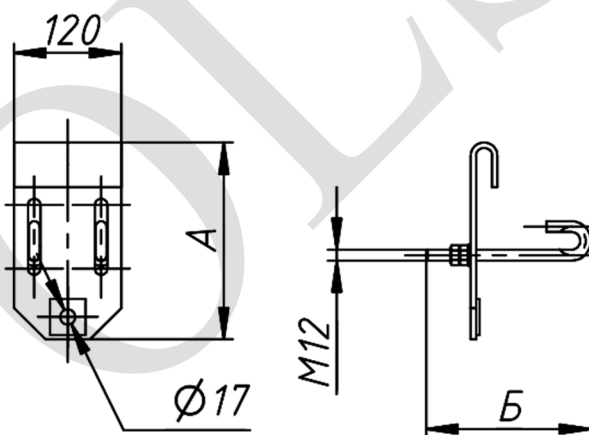
Рисунок 1. Узел крепления УТП
