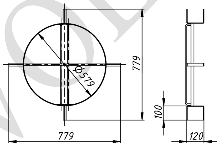
Рисунок 1. Устройство типа УПМК-08
