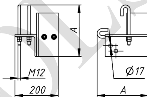
Рисунок 1. Узел натяжной УК(У)
