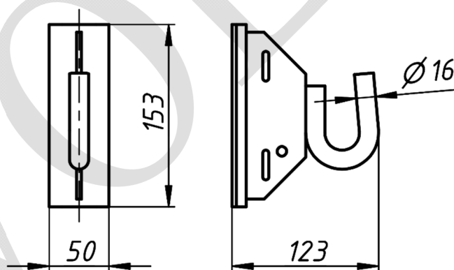
Рисунок 1. Крюк бандажный КР-16
